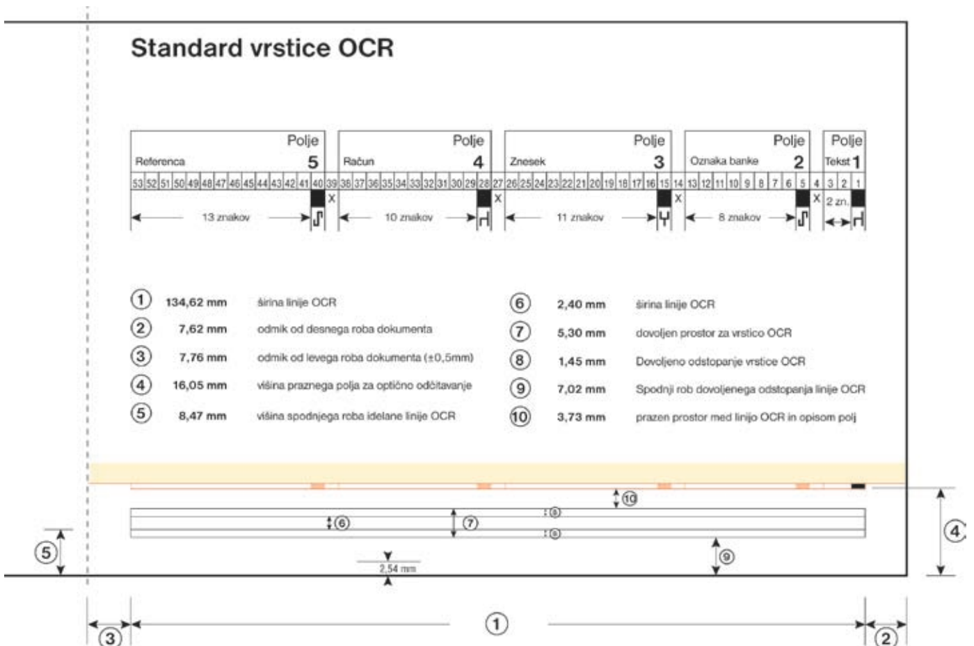
Slika 5: Standard zapisa vrstice OCR
